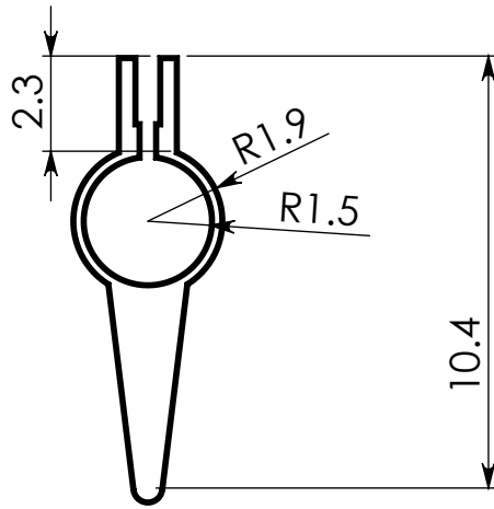
V superior
