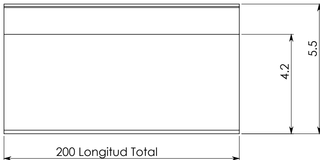
V frontal
